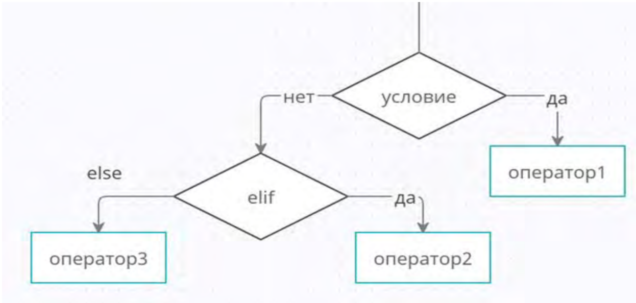
Рис. 51. Блок-схема условного оператора
